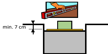
plaatsen van muurblok op egalisatielaag
