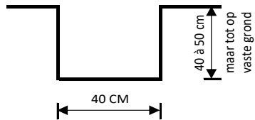
uitgraven fundering
