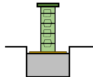
plaatsen van muurcap met betonlijm o.a. Omnicol BB of Murocol S
