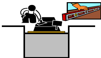
egaliseren met gebroken steenslag ± 3 cm dik
